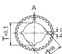
Rowek wpustowy
